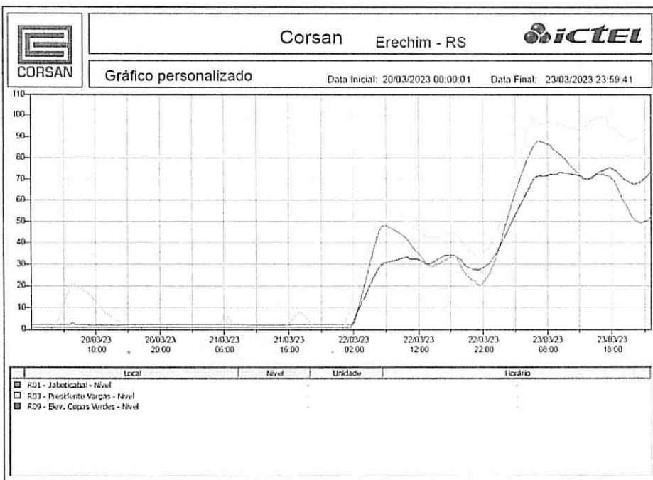
Gráfico 02: Nível dos reservatórios Jaboticabal, Presidente Vargas e Copas Verdes, de 20/03 a 23/03/23.
