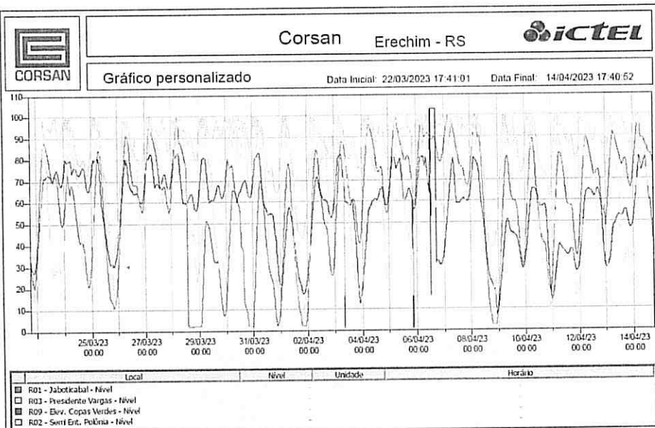
Gráfico 03: Nível dos reservatórios Jaboticabal, Presidente Vargas, Polônia e Copas Verdes, de 22/03 a 14/04/23.
