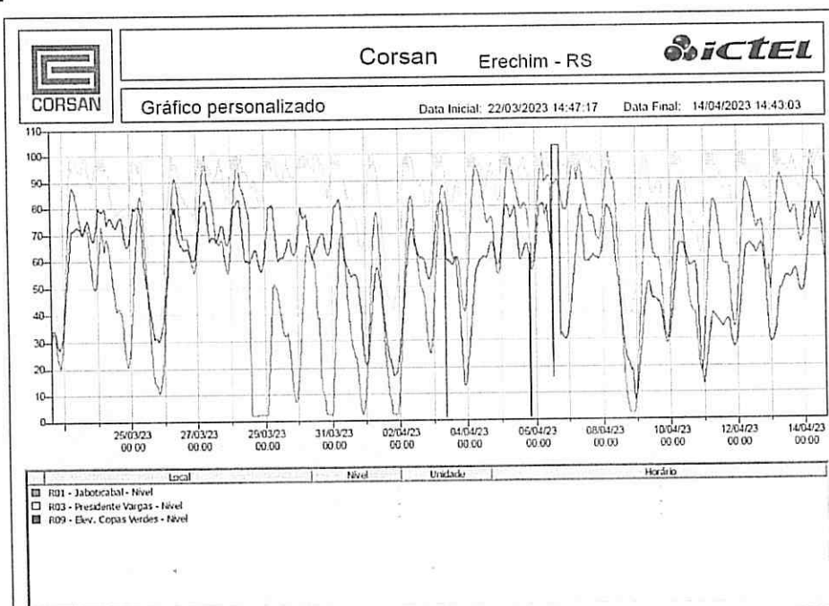
Gráfico 01: Nível dos reservatórios Jaboticabal, Presidente Vargas e Copas Verdes, de 22/03 a 14/04/23.
