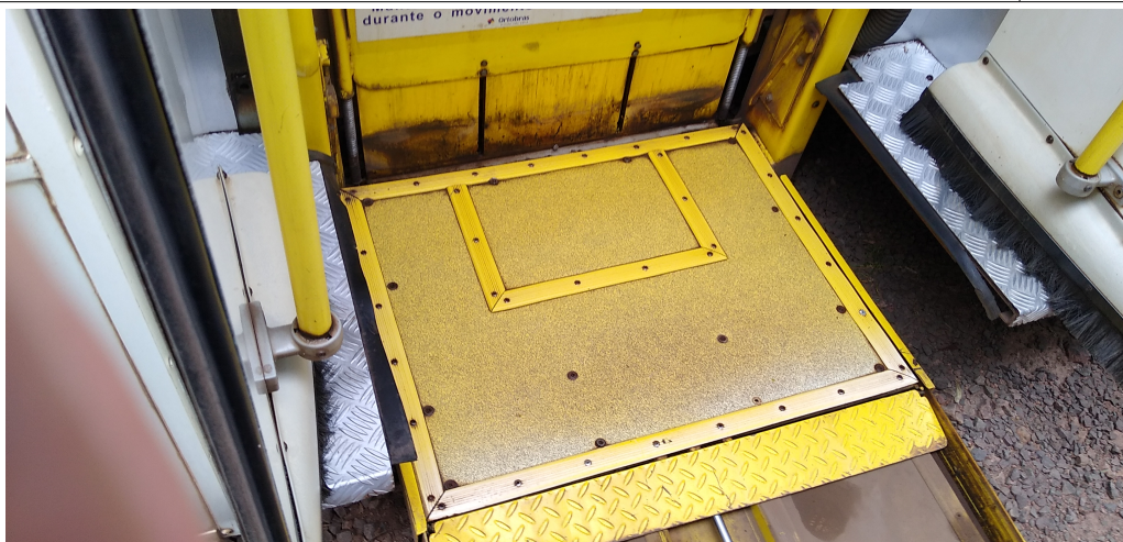
Foto 1 Plataforma Elevatória
