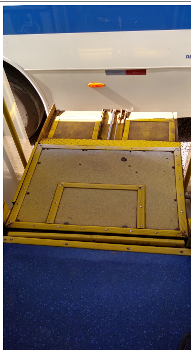
Foto 1 Plataforma Elevatória
